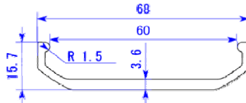
リム断面図
